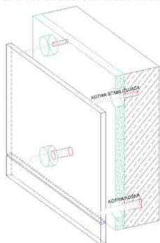
KOTWIENIE W FUDZE POZIOMEJ - KOTWY NOŚNE Z PŁASKOWNIKA
