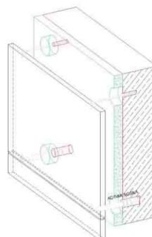
KOTWIENIE W FUDZE POZIOMEJ - KOTWY NOŚNE RUROWE
